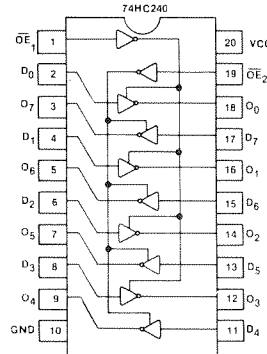
74HC240 FUNCTION TABLE
