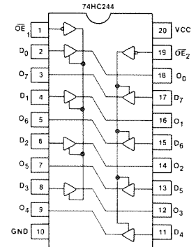
74HC244 FUNCTION TABLE
